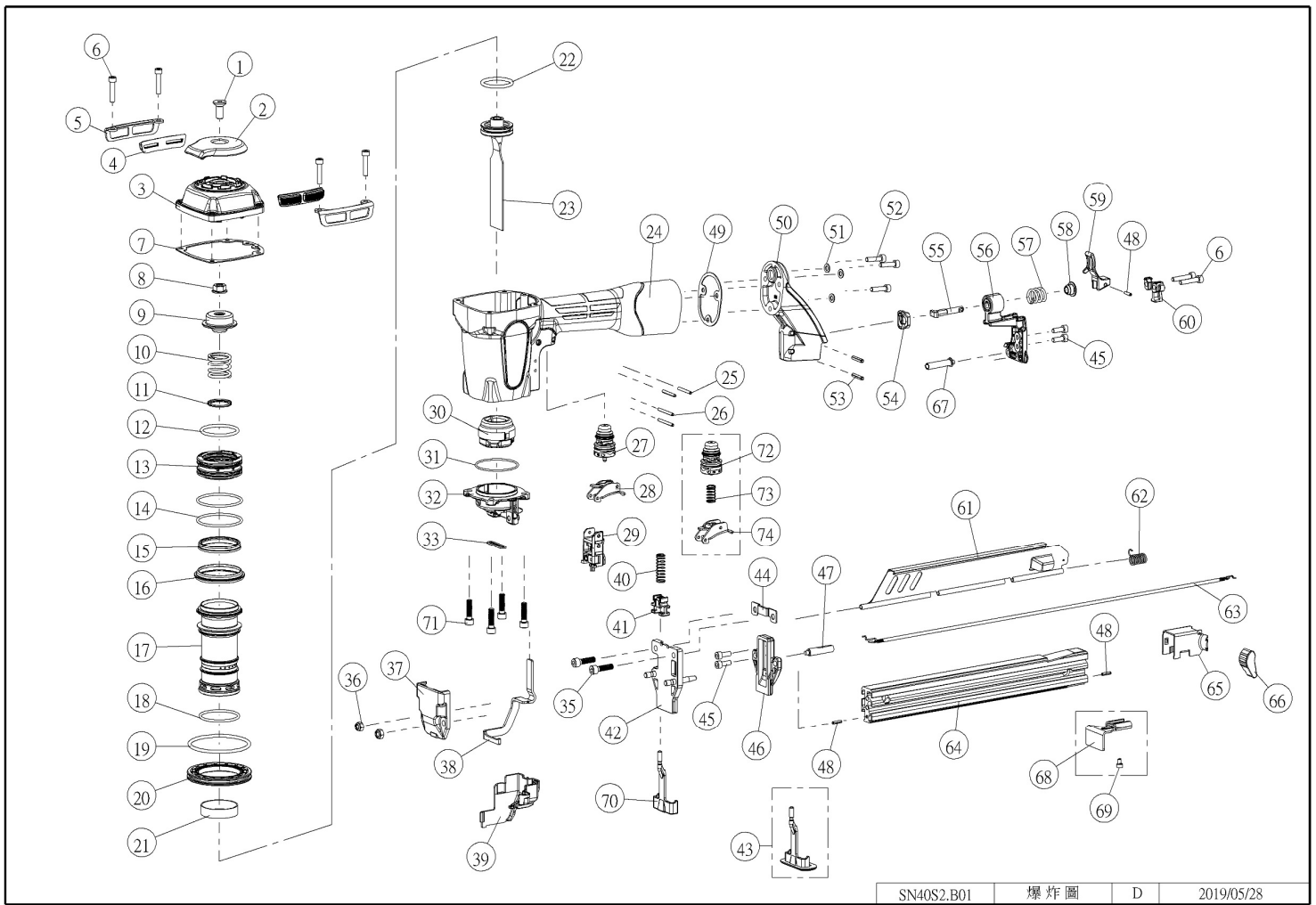
SN40S2.B01 爆炸圖 D 2019/05/28
