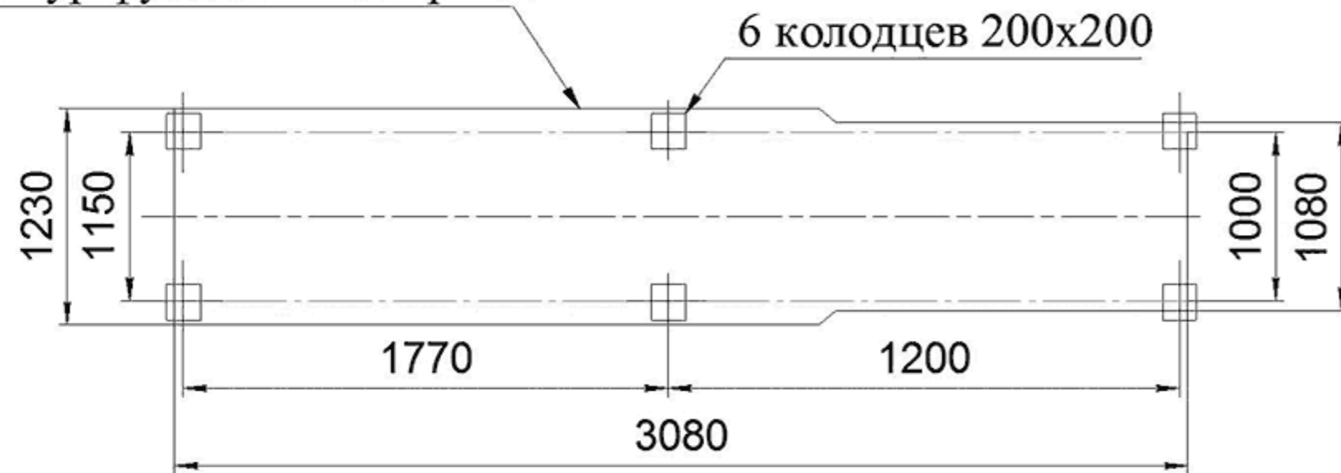
Контур фундаментной рамы
